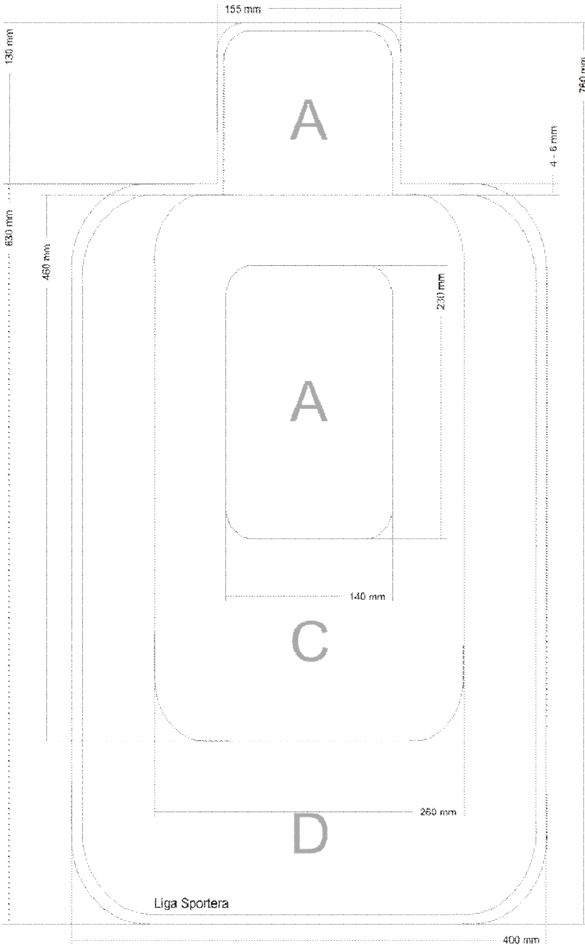
9.2.3. Tarcza Liga Sportera mini (LS mini)
