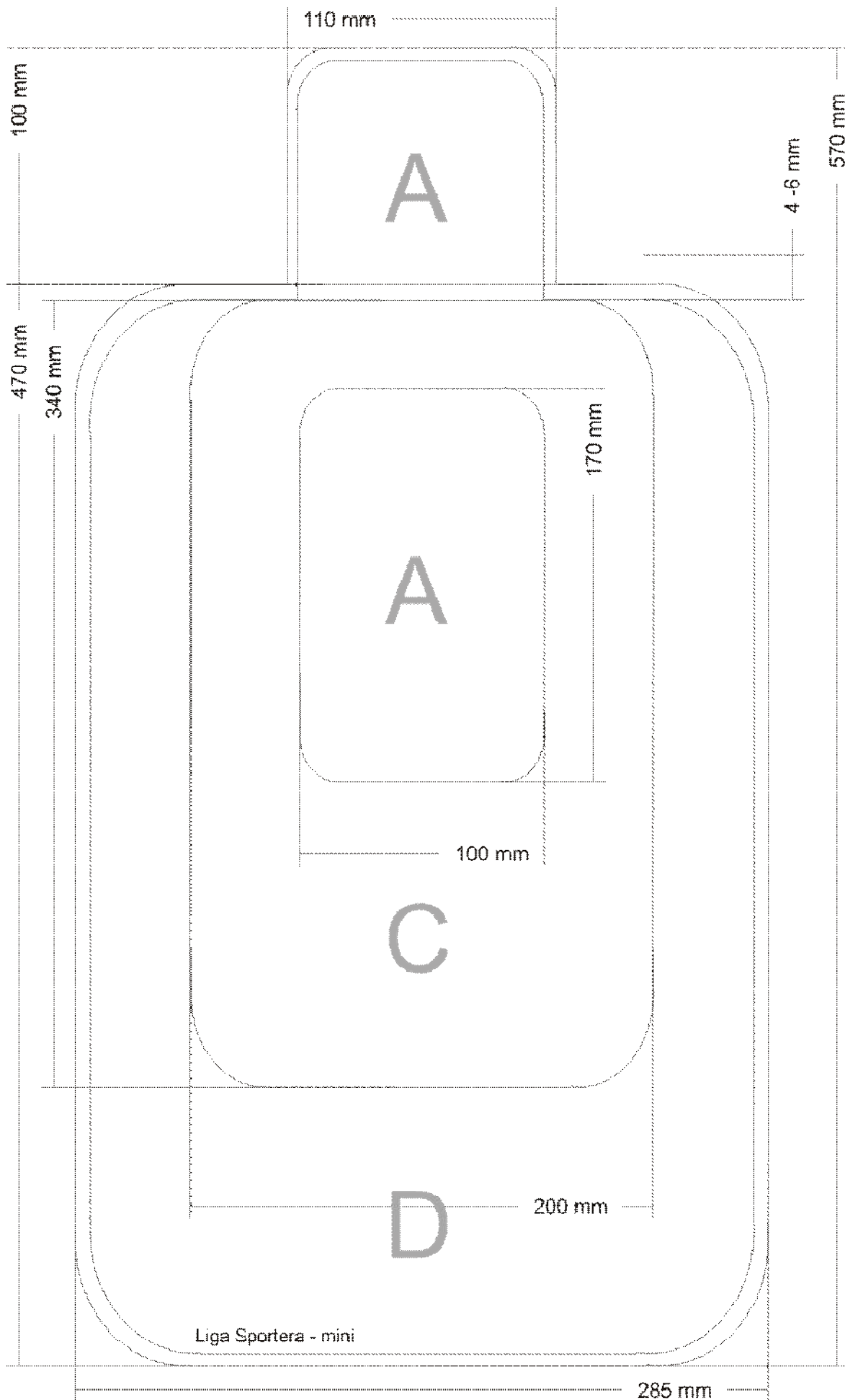
9.2.4. Tarcza Liga Sportera mikro (LS mikro)
